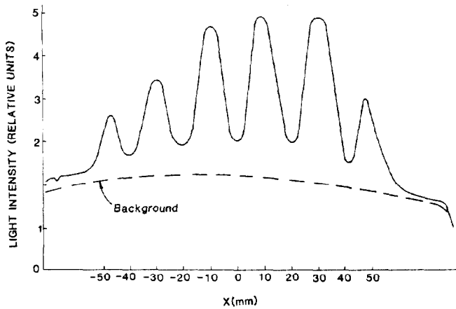
5. a. OMA emittance pattern
