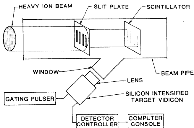
4. OMA Schematic
