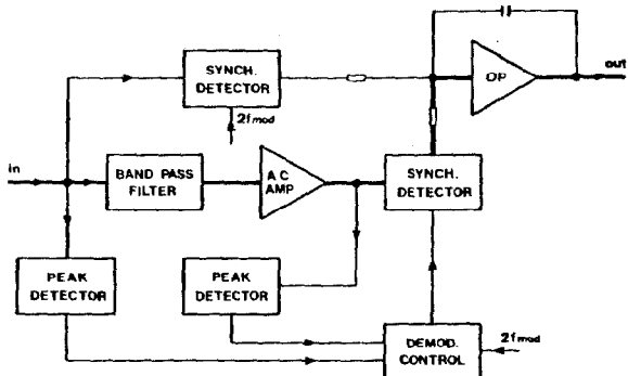
Fig. 2 - Demodulator
