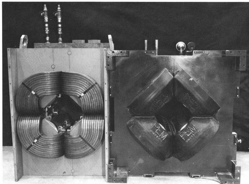
Fig. 1. 8Q16M/7 and 8Q16MK-1 quadrupole magnets
