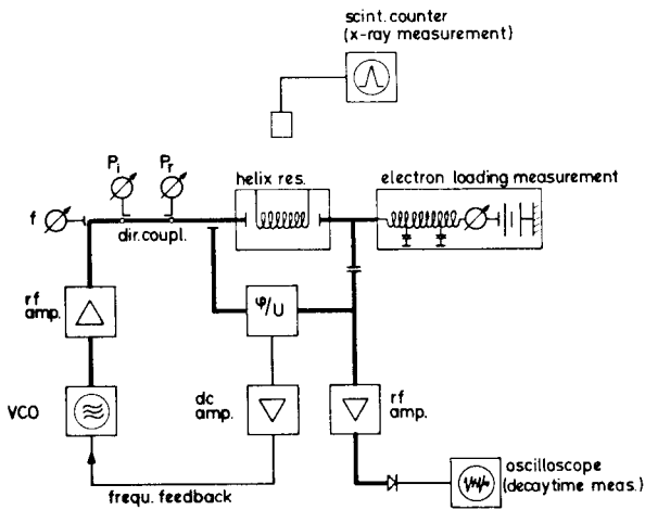
Fig. 2. Rf circuit.
